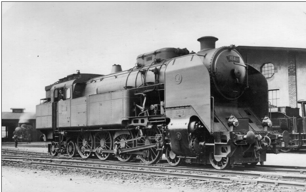
0403 ČSD 464 019 (sbírka Ing. Jindřich Rachota)
